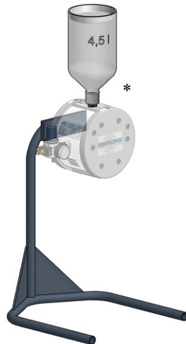
KS20850 mit Oberbehälter 4,5 Liter auf Stativ
